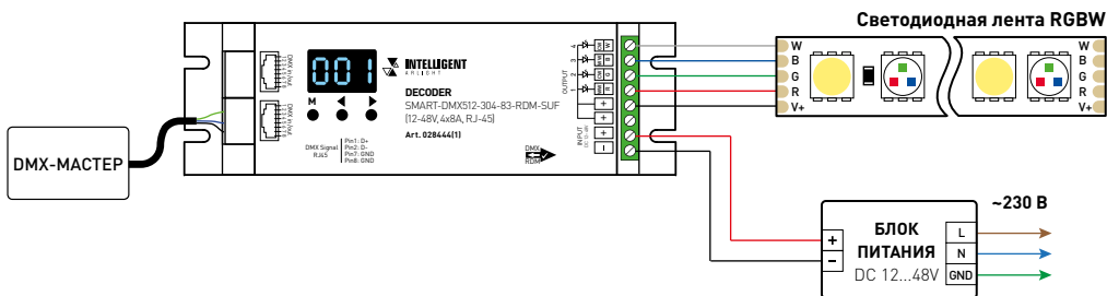
Рис. 1. Схема подключения декодера SMART-DMX512-304-83-RDM-SUF
