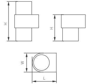
Рис. 1. Чертеж и габаритные размеры
