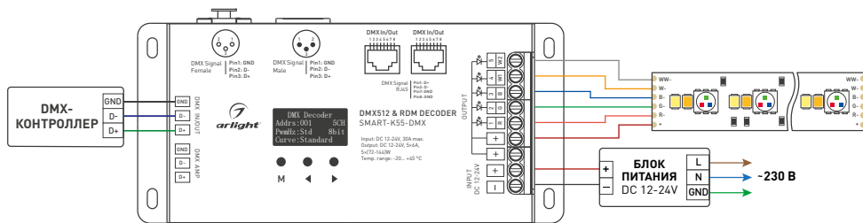
Рисунок 1. Подключение декодера SMART-K55-DMX
