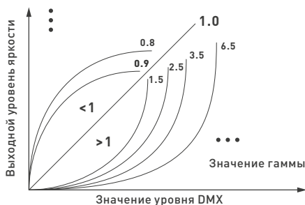
Рисунок 2. График значение гаммы
