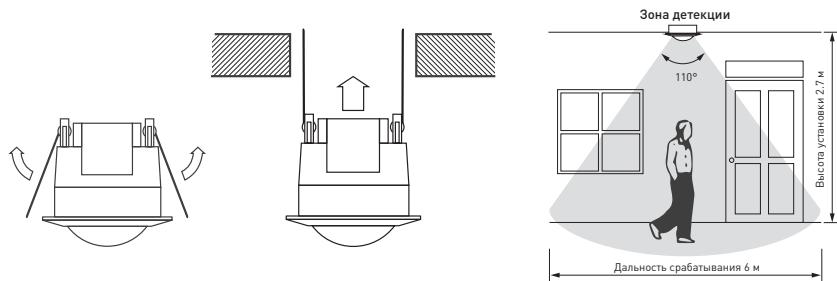
Рис. 3. Установка датчика движения
