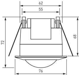
Рис. 1. Габаритный чертеж
