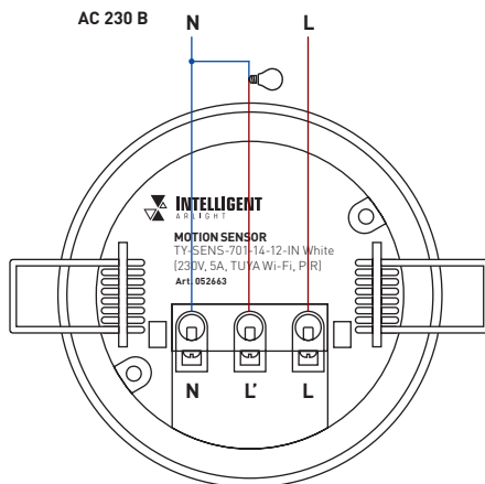
Рис. 2. Схема подключения датчика движения
