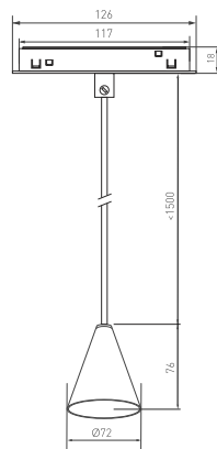
Рис. 1. Чертеж и габаритные размеры
