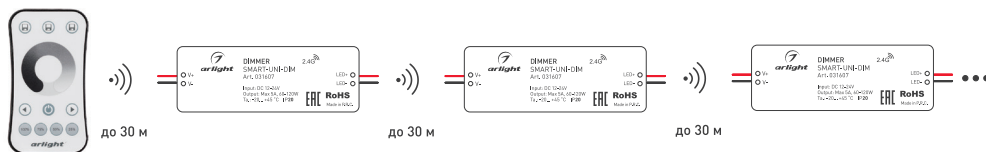
Рисунок 2. Ретрансляция сигнала от пульта ДУ [до 30 м на открытом пространстве]
