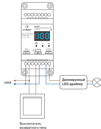
Рисунок 1 Схема подключения диммера SMART-D19-DIM-PUSH-DIM
