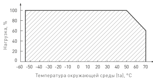
Рис. 2. Максимальная допустимая нагрузка, % от мощности источника
