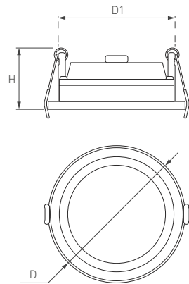
Рис. 1. Чертеж и габаритные размеры
